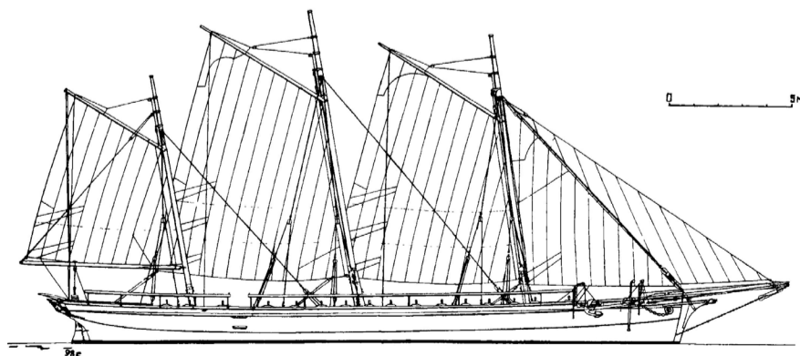
Парусно-гребная канонерская лодка, проект контр-адмирала И.И. фон Шанца, 1853 г.
